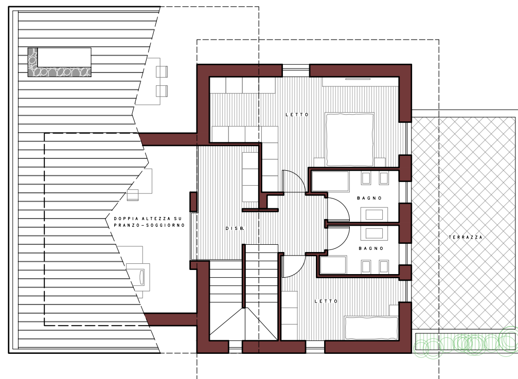
VILLA "C" PIANO PRIMO
